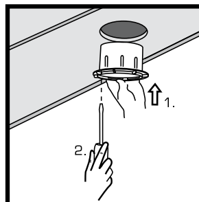
Montering av stos i undertak. Fästes med skruvar.
