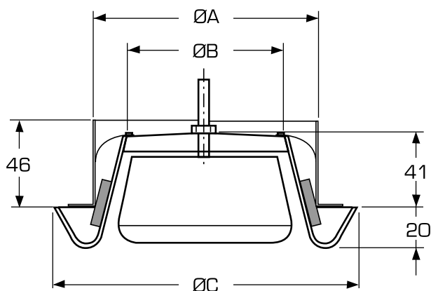
Montering av stos i vägg.
