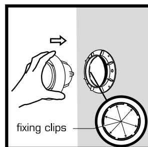
Montering av ventil i ventilstosen. Se till att någon av "ventilvingarna" bör peka mot mitten av någon låskant.
